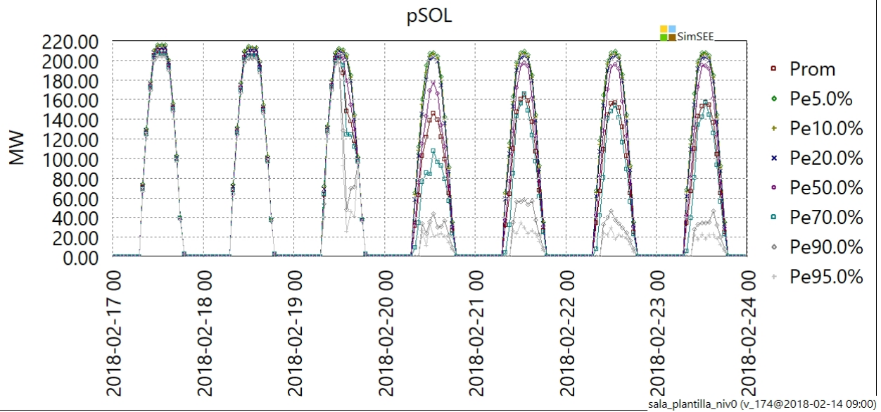
Fig 7: Generación solar.
