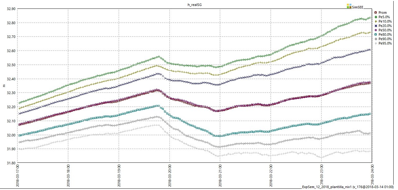
Fig 30: Operación de Salto Grande. (mitad Uruguay).
