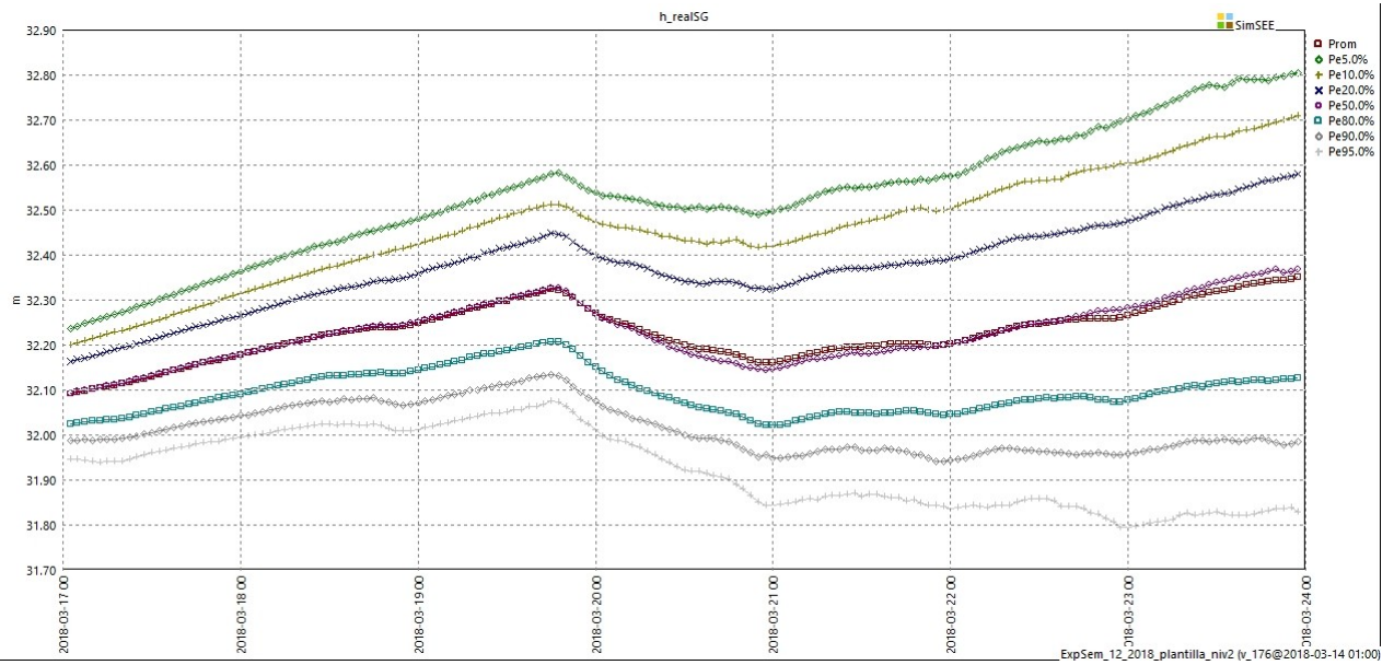
Fig 39: Operación de Salto Grande. (mitad Uruguay).
