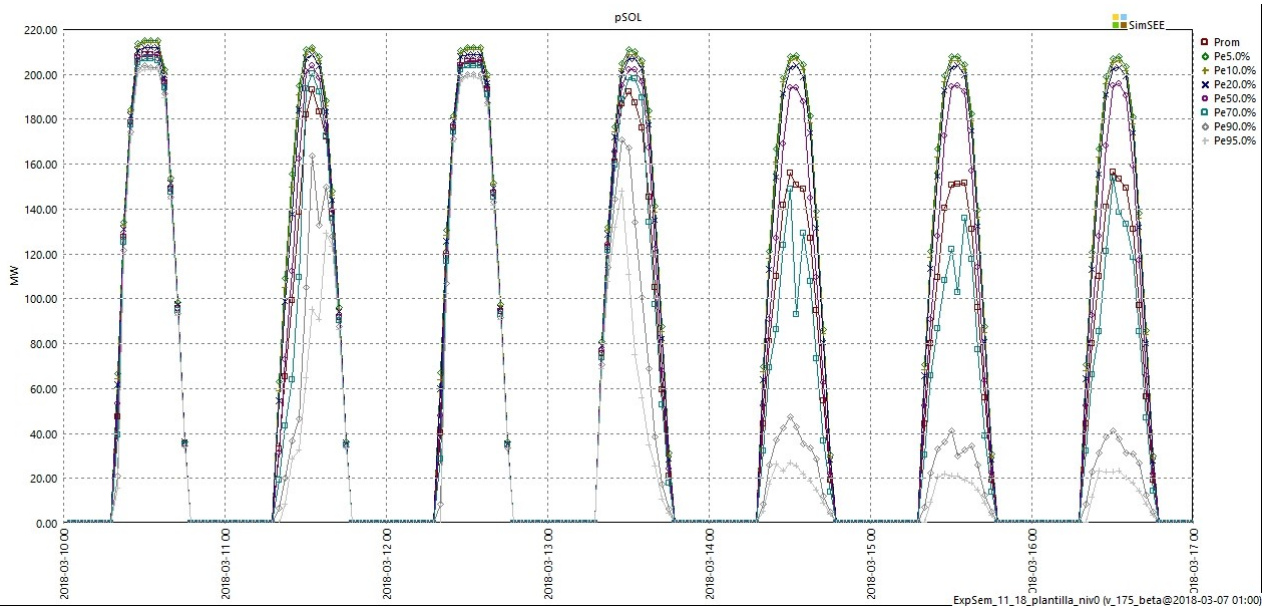
Fig 7: Generación solar.
