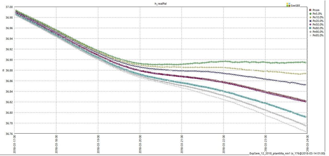
Fig 29: Operación de Palmar
