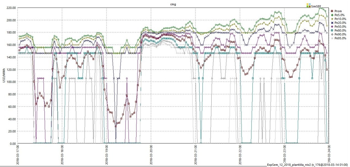
Fig 32: Costo marginal del SIN.
