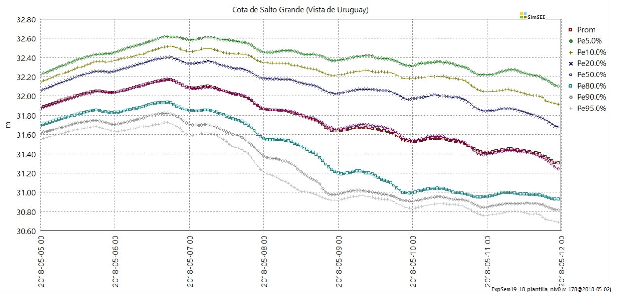
Fig 21: Operación de Salto Grande Uruguay
