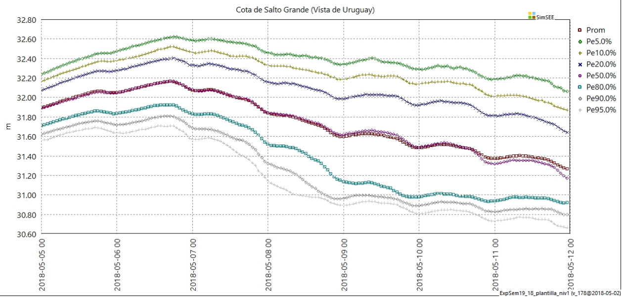
Fig 30: Operación de Salto Grande Uruguay
